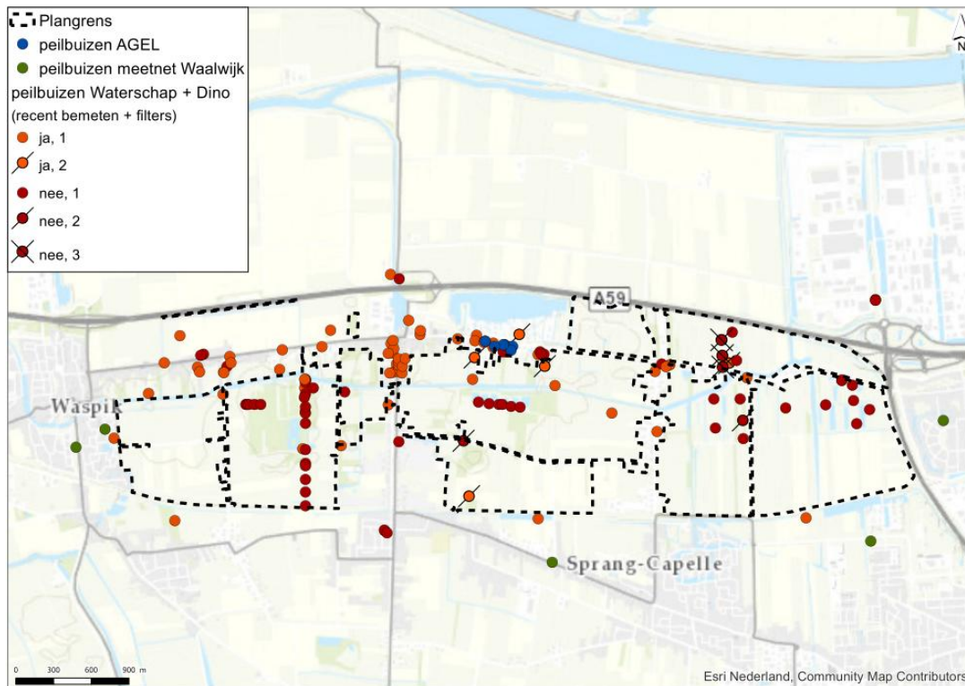
Abbeelding 3.1 Bestaande meetpunten voor het grondwater en stijghoogte in de Westelijke Langstraat
