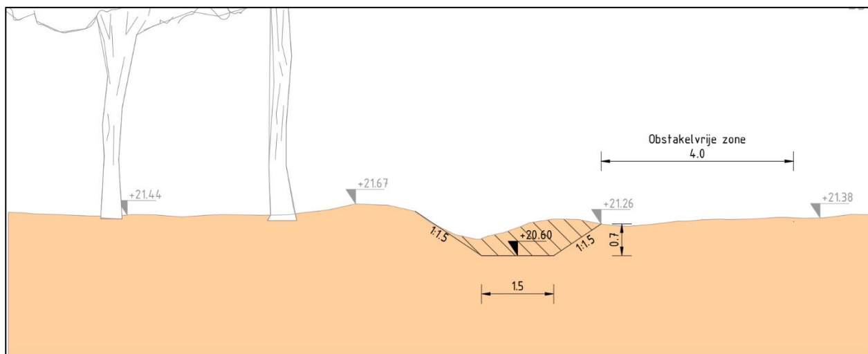
Figuur 28: Principeprofiel (P4) omleiding BZ42 & BZ57 ter hoogte van de op te waardenen OWL10825
