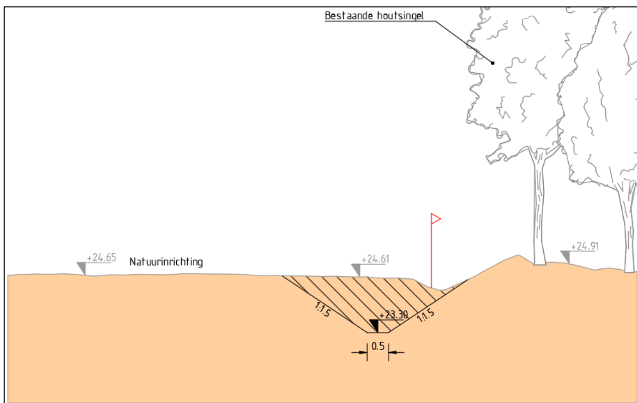
Figuur 22: Principeprofiel P2 omleiding ten zuiden van Misperleindse Heide
