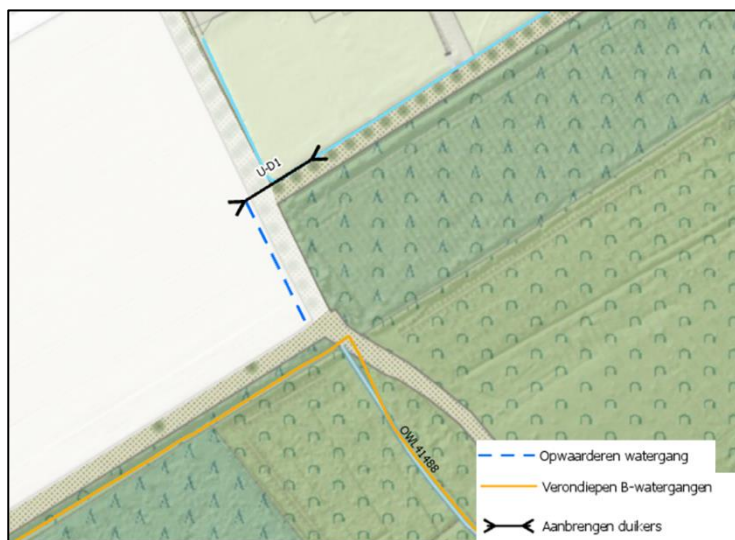
Figuur 53: Op te waarden watergang t.h.v. De Kievit inclusief aan te brengen duiker
