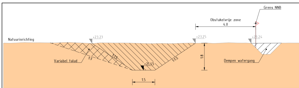
Figuur 26: Principeprofiel (P2) omleiding BZ42 & BZ57 tussen bestaande BZ42 en te dempen BERE-0329
